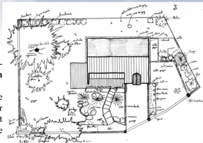
Etat existant
